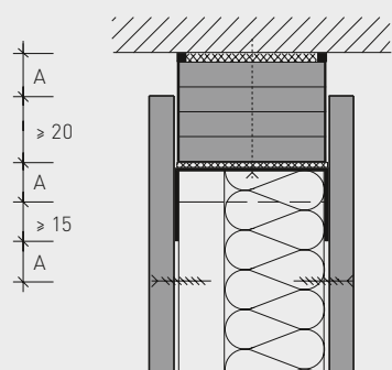
Powerpanel H 2 O-montagewand met éénlaagse beplating
