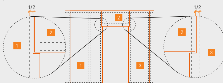
Deuropening met plaatuitspringing (variant B)
