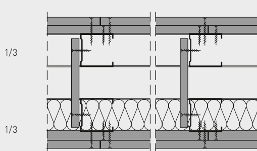
Verbinding bij een installatiewand
