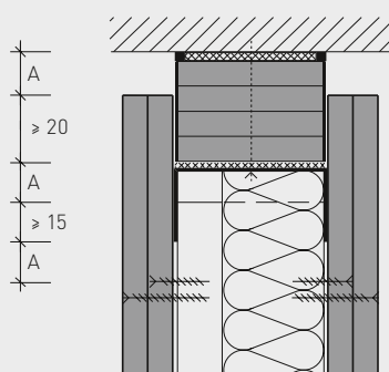
Powerpanel H 2 O-montagewand met tweelaagse beplating
