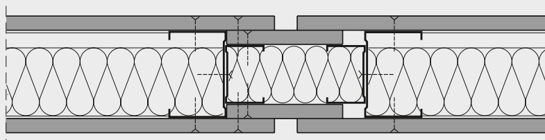
fermacell Powerpanel H 2 O-montagewand met éénlaagse beplating, dilatatievoeg met plaatstroken
