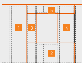
Raamopening bij horizontale beplatingsvoeg
