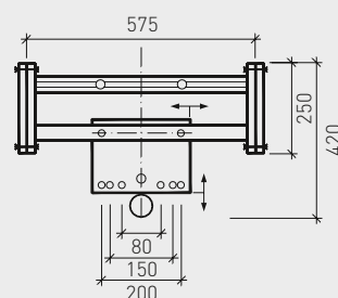
Traverse voor kleine wastafels (maten in mm)
