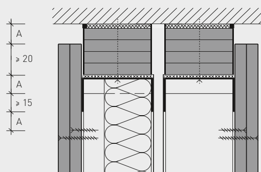
Powerpanel H 2 O-montagewand met tweelaagse beplating, uitgevoerd als een dubbele profielwand
