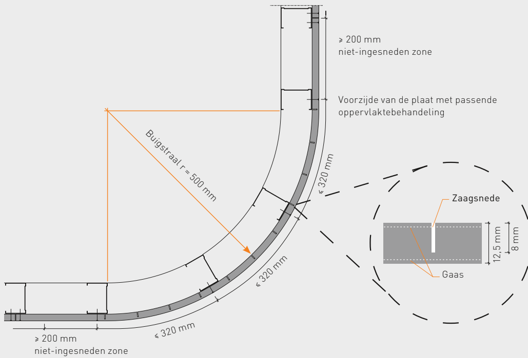
Buitenronding buigstraal r = 500 mm
