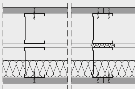
Powerpanel H 2 O-montagewand zonder en met geïsoleerde holle ruimte, uitgevoerd als dubbele staanderwand met éénlaagse beplating. CW-profielen los van elkaar geplaatst (links) of verbonden door zelfklevende cellenband (rechts).
