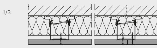
Onderconstructie uit CW-profiel met verende aanpasbeugel, éénlaagse beplating
