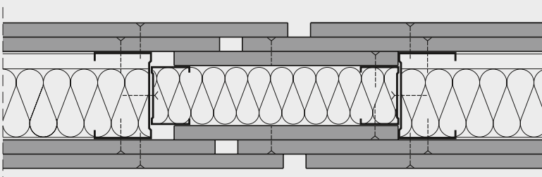
fermacell Powerpanel H 2 O-montagewand met tweelaagse beplating, dilatatievoeg met plaatstroken
