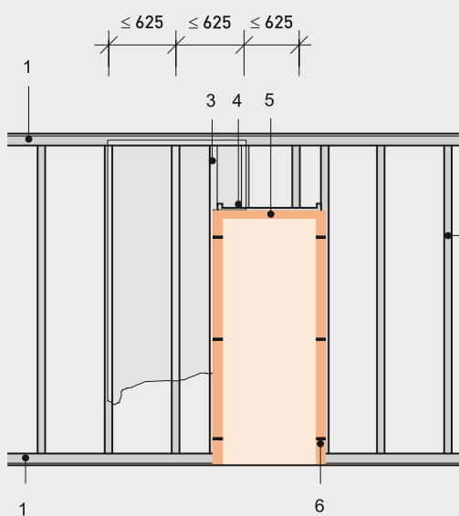
Inbouwschema van het kozijn met onderconstructie (maten in mm)
